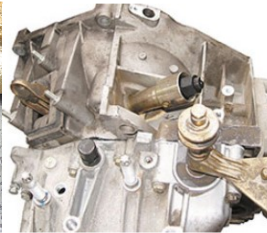
Ειδικό εργαλείο αφαίρεσης του δίχαλου.
